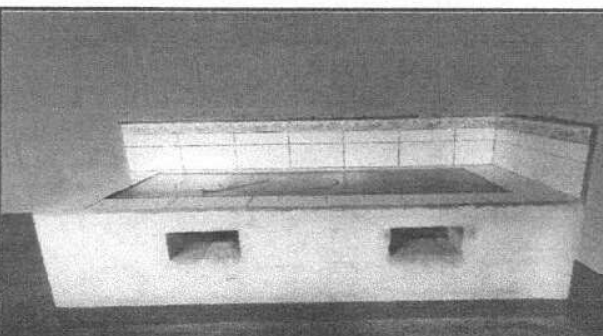
Foto 6: MODULO 3. CONSTRUCCION E INSTALACION DE AZULEJO EN ESTUFA RURAL.
